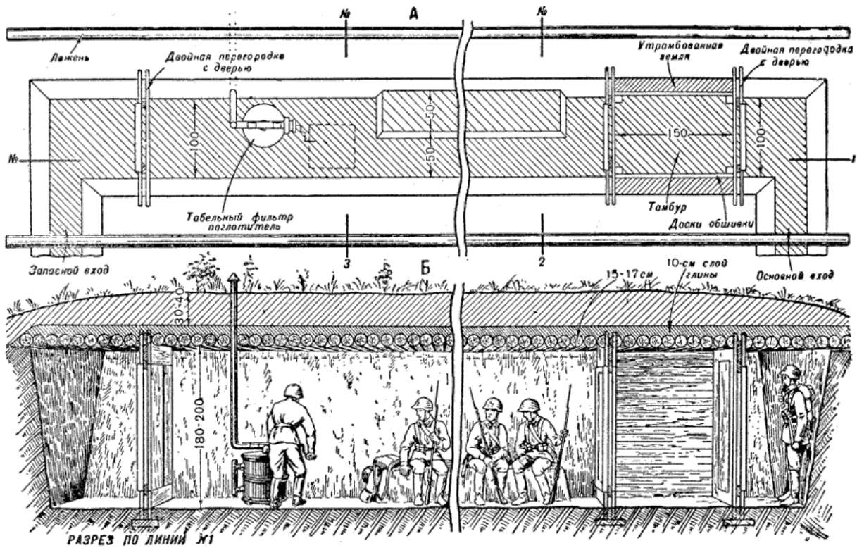
РАЗРЕЗ ПО ЛИНИИ X1
