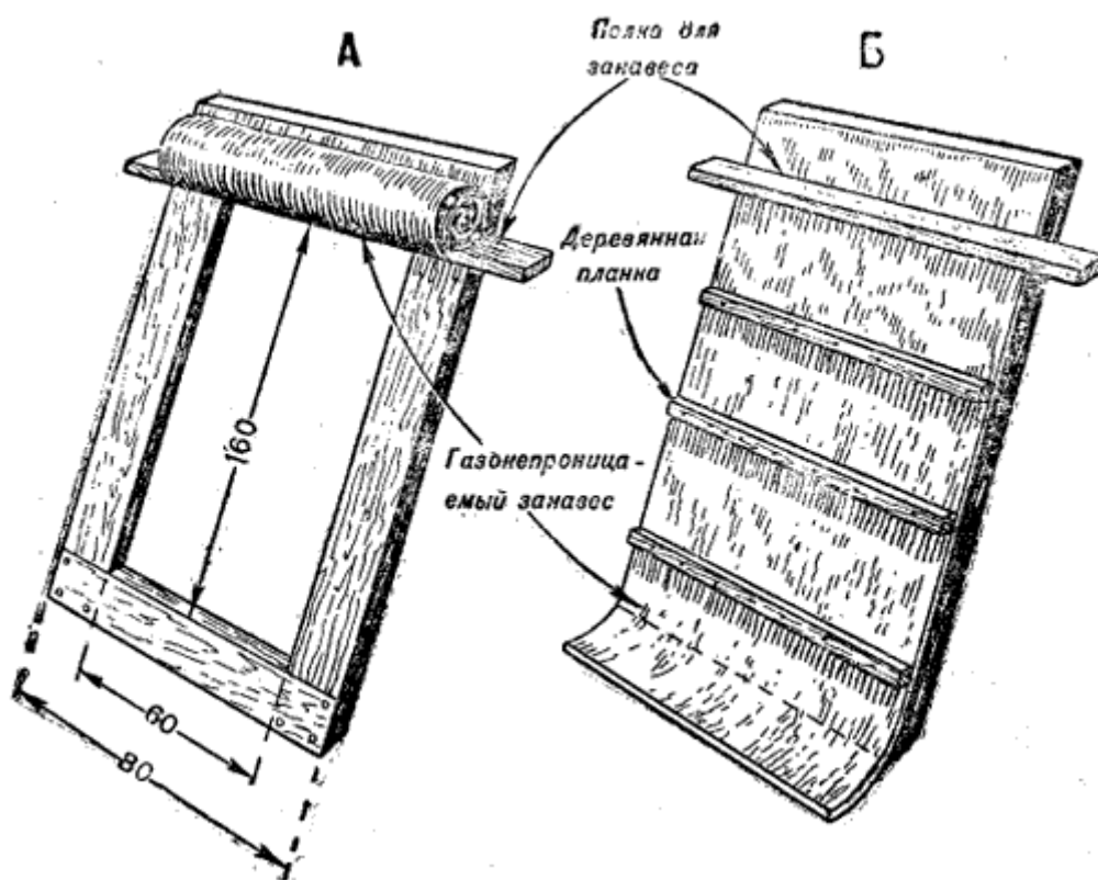
Рис. 86. Устройство газонепроницаемого занавеса: А - занавес открыт; Б - занавес закрыт
