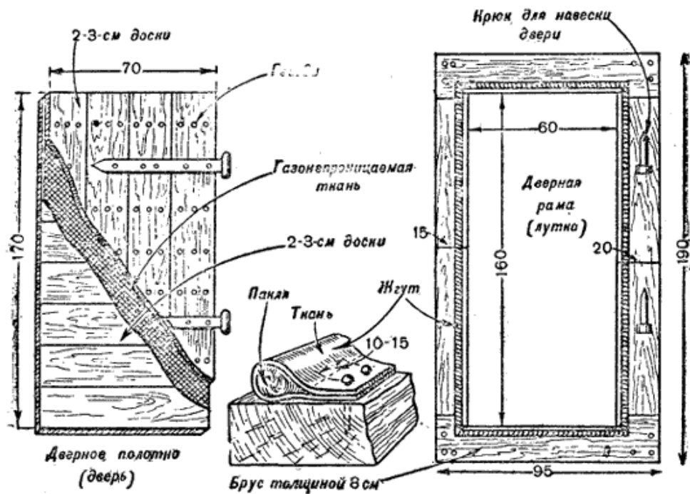
Рис. 84. Устройство герметичной (газонепроницаемой) двери
