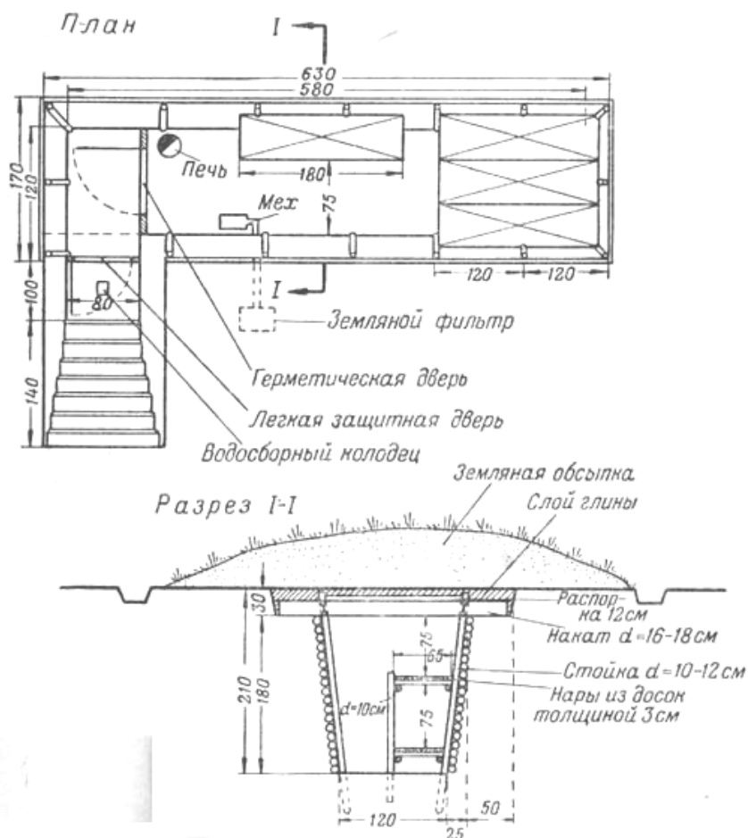
Рис. 26. Схемы землянок-укрытий: а — на 10 человек; б — на 7 человек
