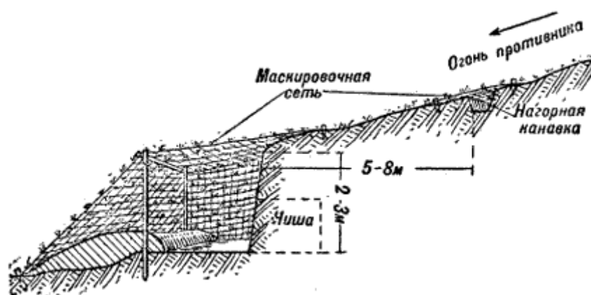
Рис. 79. Открытый заслон
